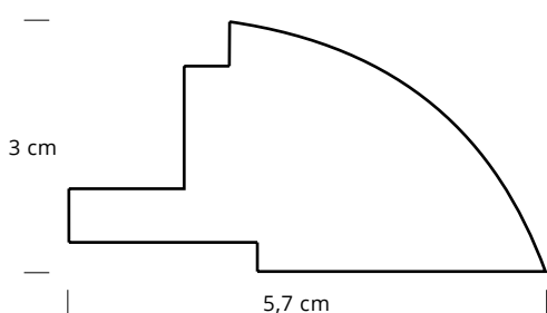
Sezione cornici scala 1:1 Frames section scale 1:1
