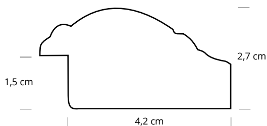
Sezione cornice scala 1:1 Frame section scale 1:1
