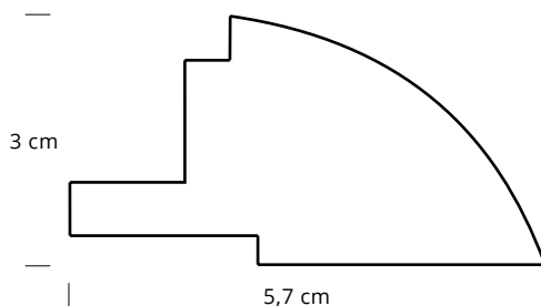
CNR 2140 PTC cornice - frame 37,5x32,5 cm ceramica - ceramic 21x16 targa - plaque 11x16 cm (cornice senza vetro - frame without glass)
