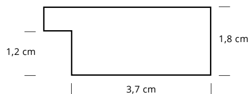
Sezione cornice scala 1:1 Frame section scale 1:1
