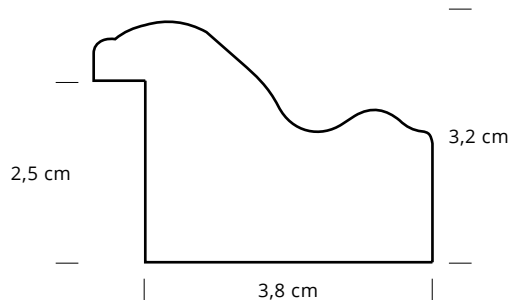
CNR 2300 RR Pass singolo raso rosso
