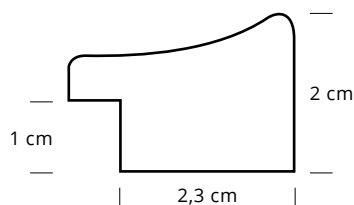
Sezione cornice scala 1:1 Frame section scale 1:1
