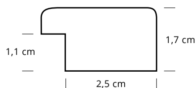
Sezione cornice scala 1:1 Frame section scale 1:1
