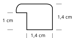
Sezione cornice scala 1:1 Frame section scale 1:1
