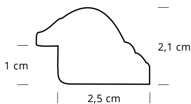
Sezione cornice scala 1:1 Frame section scale 1:1
